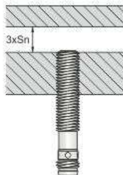
Montaje enrasado
